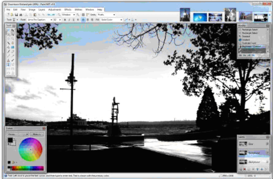
Captura pant-1
